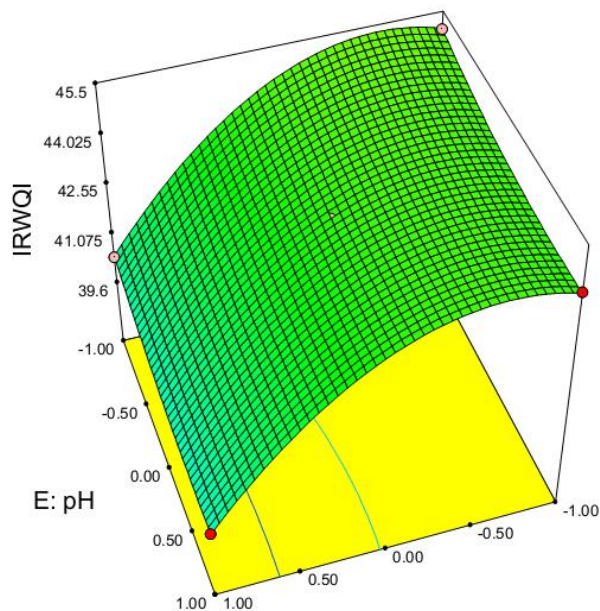
Fig. 11- Effects of pH and phosphate on IRWQI Sc شکل ۱۱- تأثیر پارامترهای pH و فسفات بر مقدار IRWQI Sc
