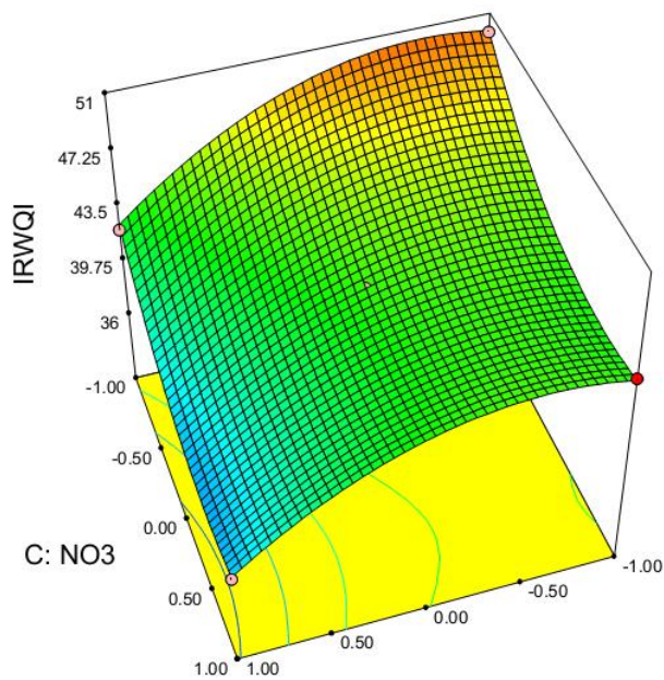
Fig. 10- Effects of nitrate and EC on IRWQI Sc شکل ۱۰- تأثیر پارامترهای نیترات و EC بر مقدار IRWQI Sc
