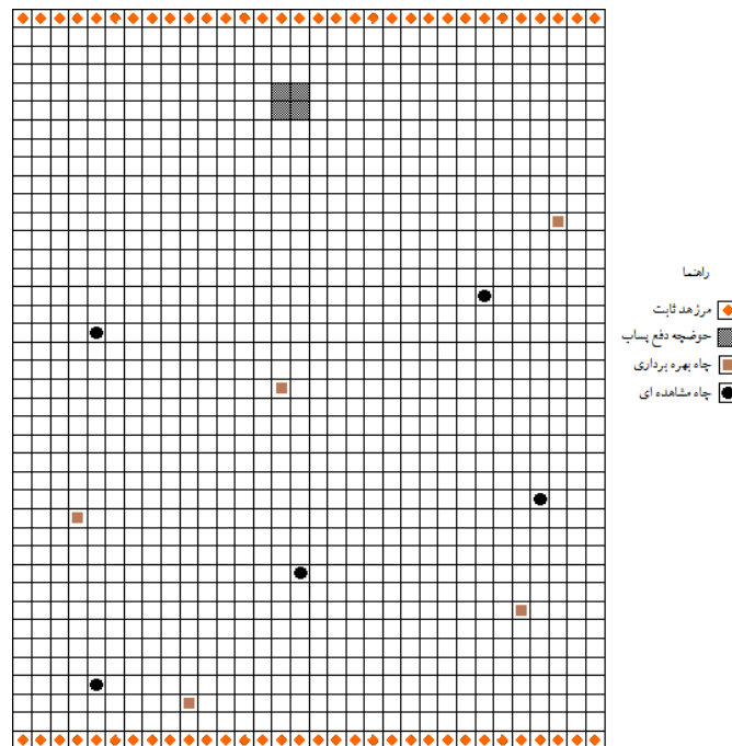
شکل ۱ - مشخصات و شبکه مدل عددی محدوده مطالعاتی برای شبیه سازی حرکت و غلظت آلودگی آب زیرزمینی
