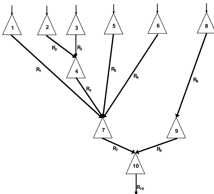
شکل ۳- مسأله بهره برداری از سیستم ده مخزنه (جلالی، ۱۳۸۴)
