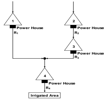
شکل ۲ - مسئله بهره برداری از سیستم چهار مخزنه (جلالی، ۱۳۸۴)
