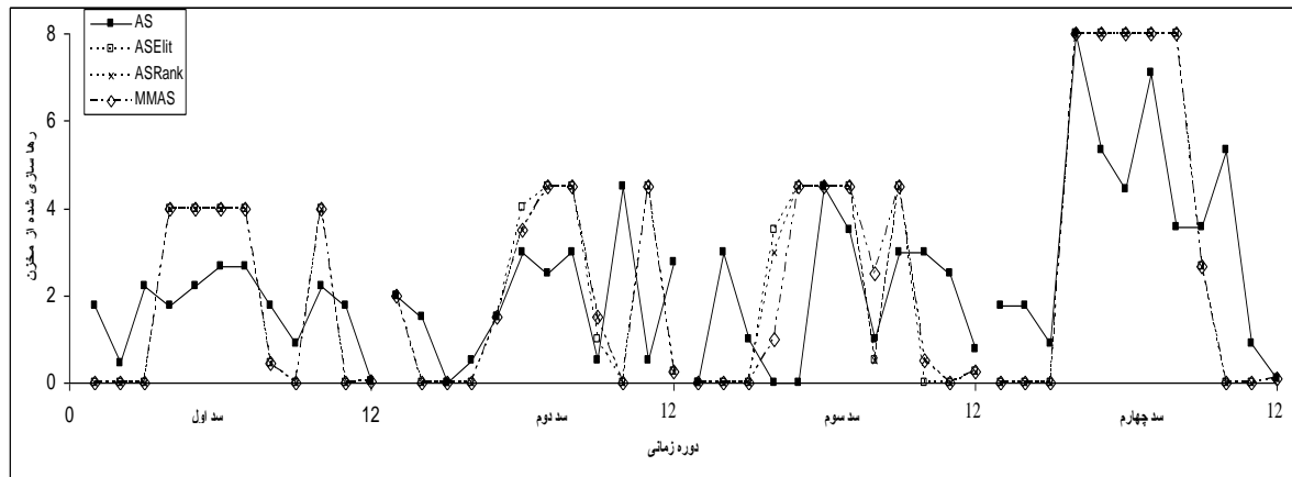
شکل ۵- مقدار بهینه آب رها سازی شده از مخازن با استفاده از فرمول بندی I الگوریتم سیستم مورچه پیشینه-کمینه در مسأله چهار مخزنه
