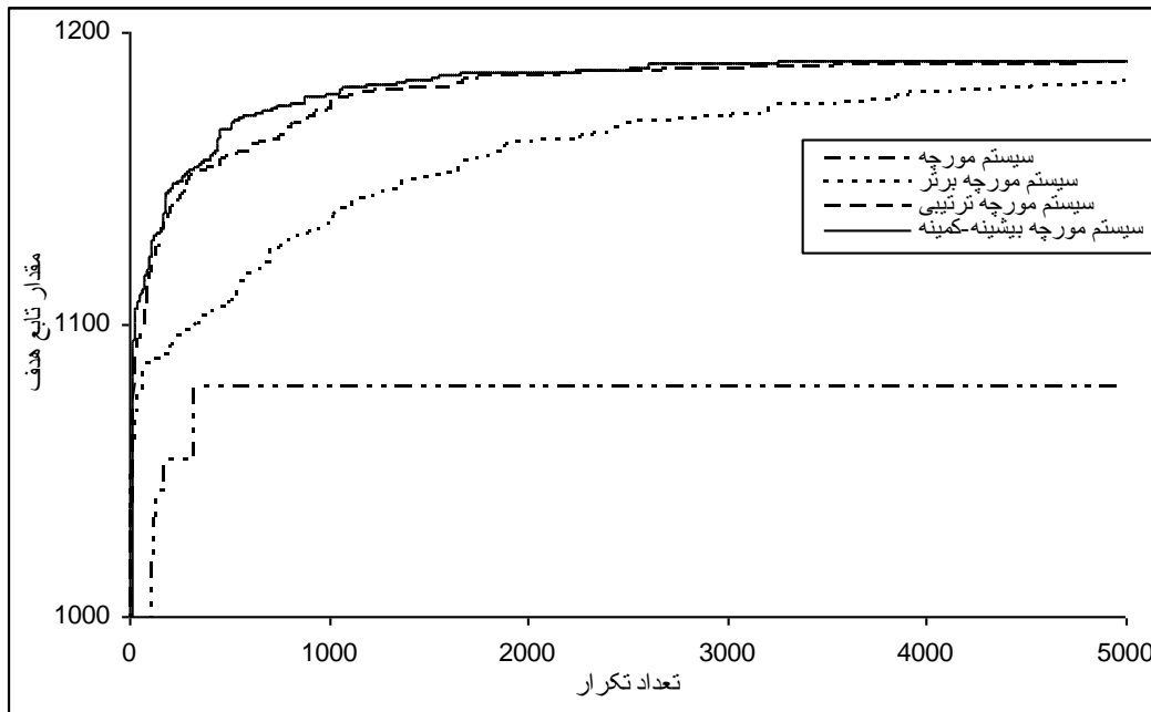
شکل ۹- نحوه همگرایی حداکثر مقدار تابع هدف مسأله با استفاده از فرمولبندی I الگوریتم‌های مختلف پیشنهادی در مسأله چهار مخزنه
