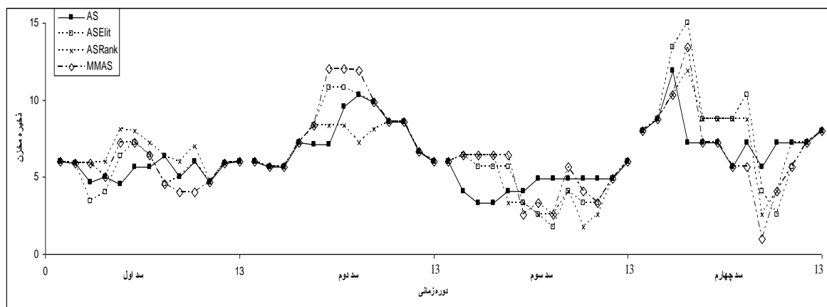
شکل ۶- مقدار بهینه ذخیره مخازن با استفاده از فرمول بندی II الگوریتم سیستم مورچه پیشینه-کمینه در مسأله چهار مخزنه
