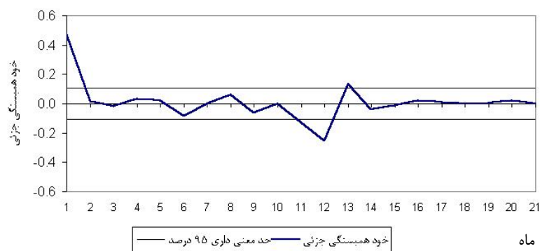
شکل ۵- تابع خود همبستگی تفاضلی جزئی فصلی رواناب ماهانه ایستگاه هیدرومتری چم چیت
