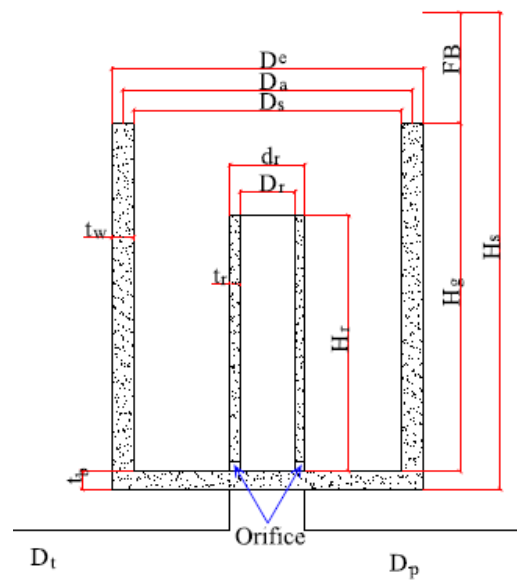
شکل ۲- جزئیات سازه ای یک مخزن موجگیر دیفرانسیل
