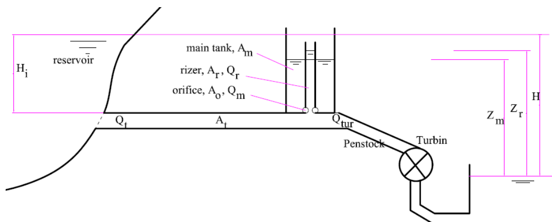
شکل ۱- طرح شماتیک مخزن موجگیر دیفرانسیل
