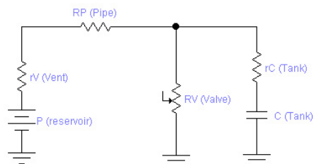
شکل ۱۵- مخزن نوع ساده، لوله و شیر
