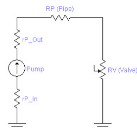
شکل ۱۶- پمپاژ از سطح آزاد
