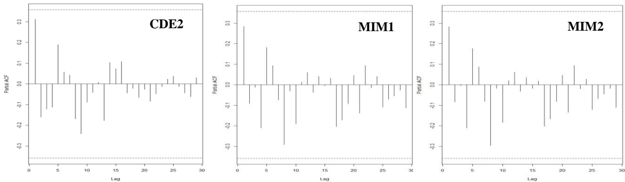
Fig. 4. ACF and PACf for CDE2, MIM1 and MIM2 models for exploring the number of p in AR (p) model شکل ۴- نمودار PACF برای شناسایی عدد p در مدل AR(p) برای مدل های CDE2 و MIM1 ، MIM2
