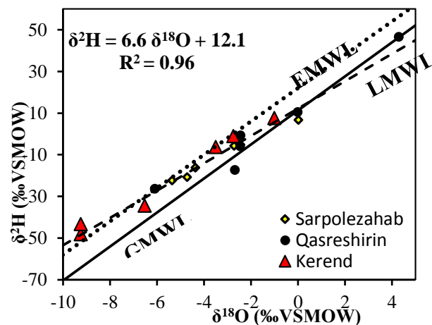
Fig. 2- Plotted rain water samples on \delta^2\text{H} vs. \delta^{18}\text{O} diagram and local meteoric water line شکل ۲- موقعیت نمونه‌های آب باران بر روی نمودار پراکنش \delta^2\text{H} در مقابل \delta^{18}\text{O} و خط آب جوی محلی
