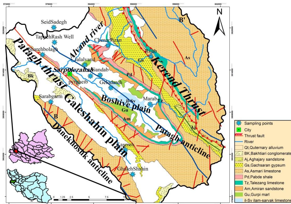
Fig. 1- Geological map of Sarpolzahab area and the sampling points شکل ۱- نقشه زمین‌شناسی محدوده مطالعاتی پل‌ذهاب و نقاط نمونه‌برداری
