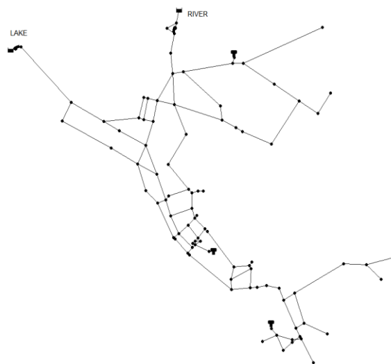
Fig. 1- Schematic representation of water distribution network of example 3 in EPANET 2.0 شکل ۱- نمایش شماتیک شبکه توزیع آب مثال ۳ نرم‌افزار EPANET 2.0
