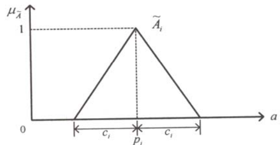
شکل ۴- تابع عضویت ضرایب فازی
