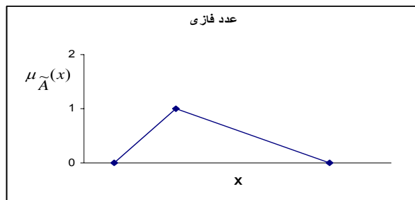
شکل ۳- عددی فازی \tilde{A}
