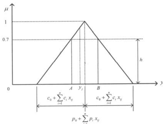
شکل ۵- تابع عضویت خروجی فازی
