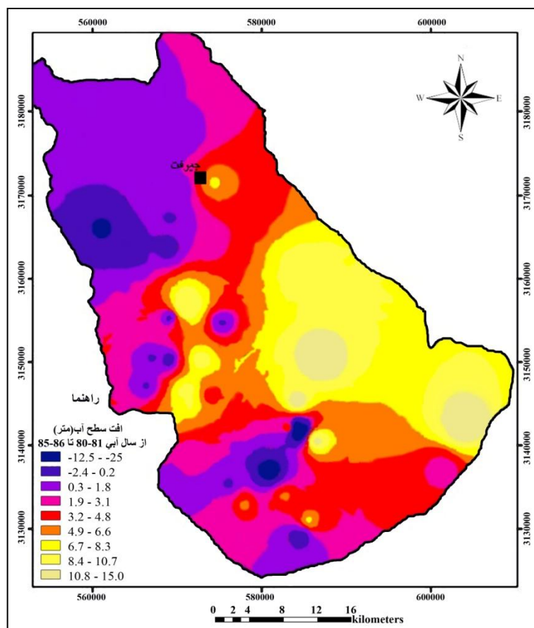
شکل ۲- نقشه افت سطح آب زیرزمینی از سال ۱۳۸۰-۸۱ تا ۱۳۸۵-۸۶
