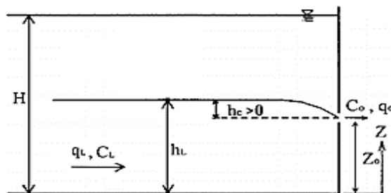
شکل ۴- پارامترهای جریان غلیظ در برخورد با دریاچه تخلیه کننده
