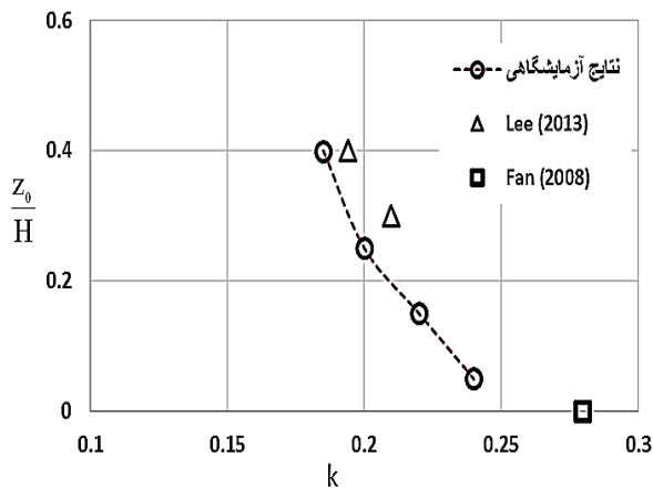
شکل ۸- تغییرات ضریب k در معادله ۴ نسبت به موقعیت‌های دریچه تخلیه کننده
