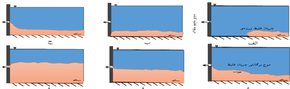
شکل ۳- تغییرات زمانی نحوه برخورد جریان غلیظ به دیواره و تخلیه آن از دریچه
