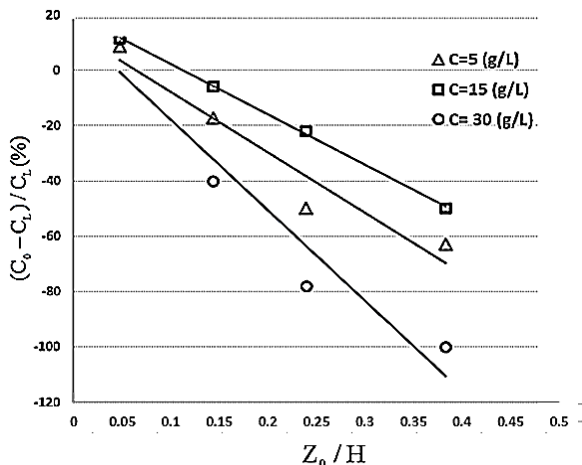
شکل ۶- درصد کاهش نسبی غلظت جریان غلیظ خروجی نسبت به موقعیت‌های دریاچه تخلیه کننده
