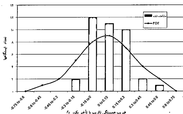
شکل ۵- مقایسه هیستوگرام r_1 و تابع چگالی احتمال حوزه آبریز کرخه
