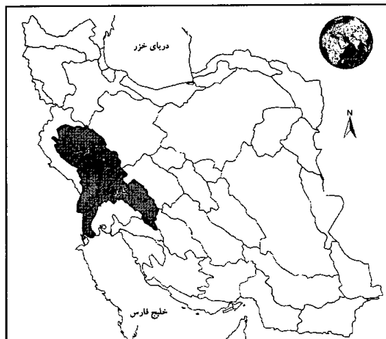
شکل ۱- موقعیت حوزه‌های آبریز کرخه، دز و کارون در ایران
