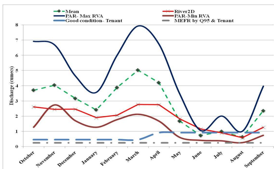
Fig. 5- Comparing parametric RVA results with River2D, Tenant and Q95 methods شکل ۵- مقایسه نتایج پارامتری RVA با روش‌های River2D، تنانت و Q95
