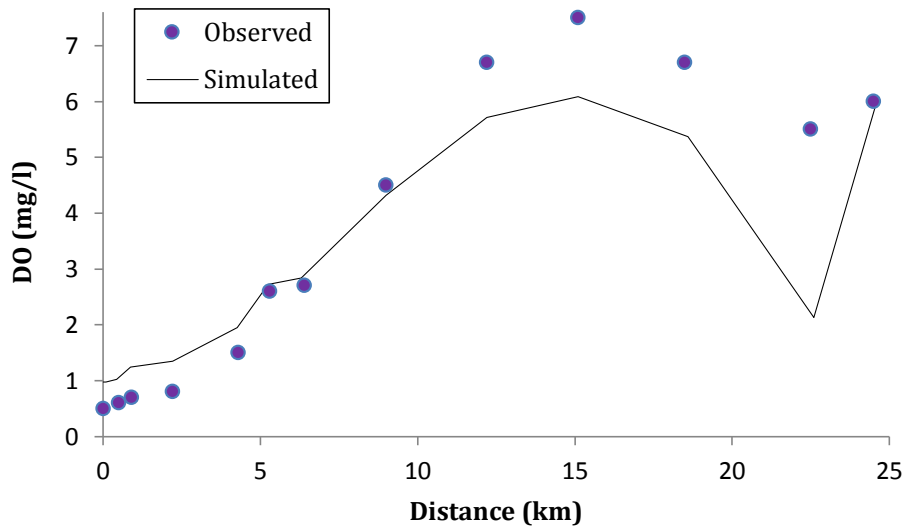
Fig. 2- DO variation along Zarjub River شکل ۲- تغییرات DO در طول رودخانه زرچوب
